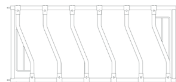
DeLaval foderfront FF60 med DS
