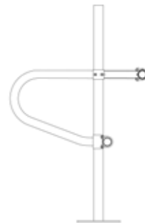
DeLaval foderfront FT50 med ätbåsavskiljare
