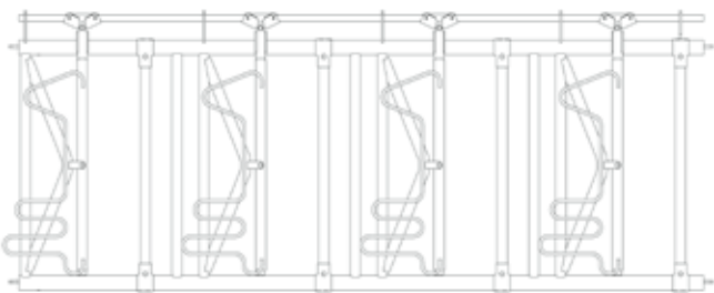
DeLaval säkerhetsfront HLS50
