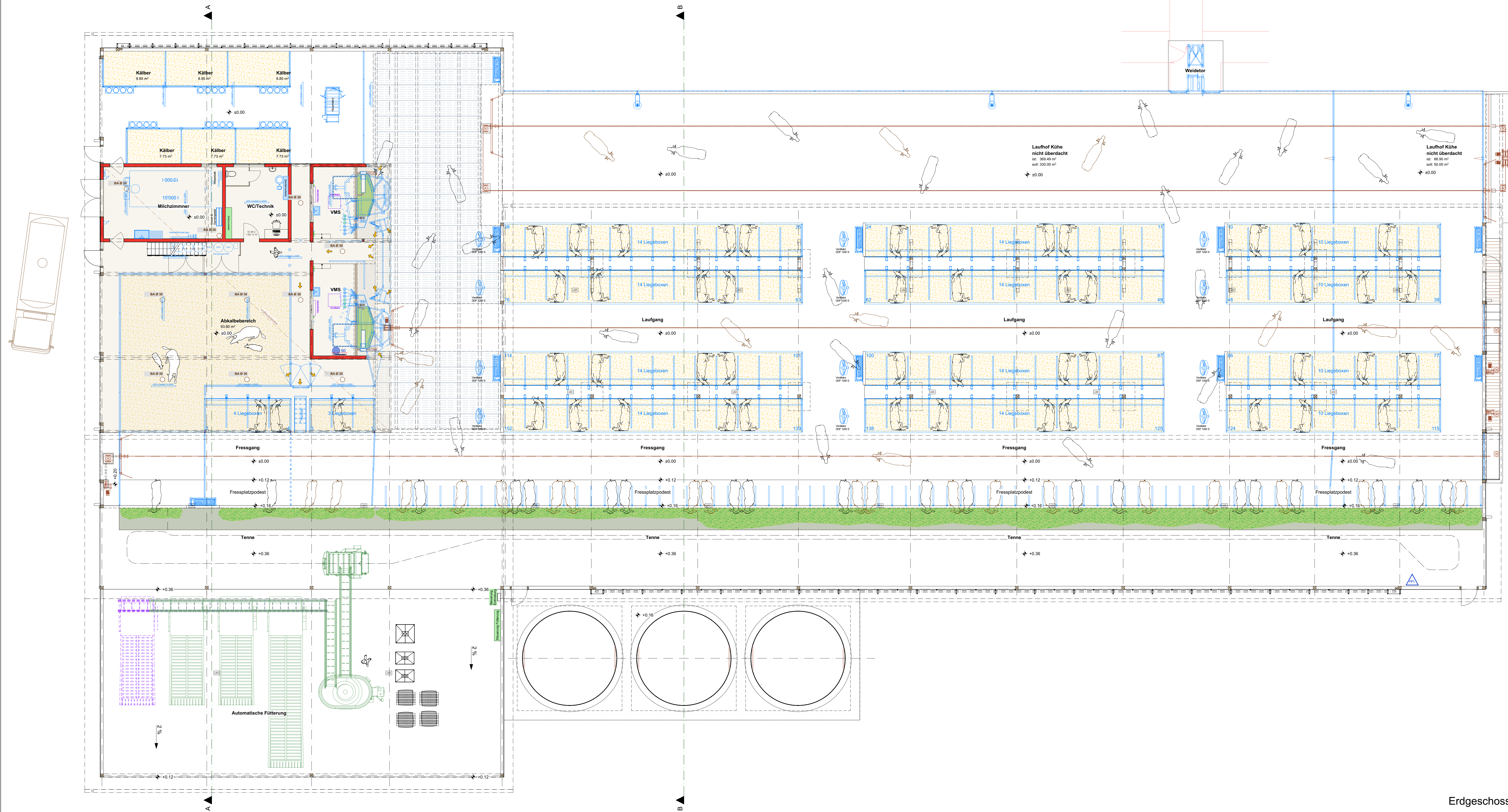
Erdgeschoss
