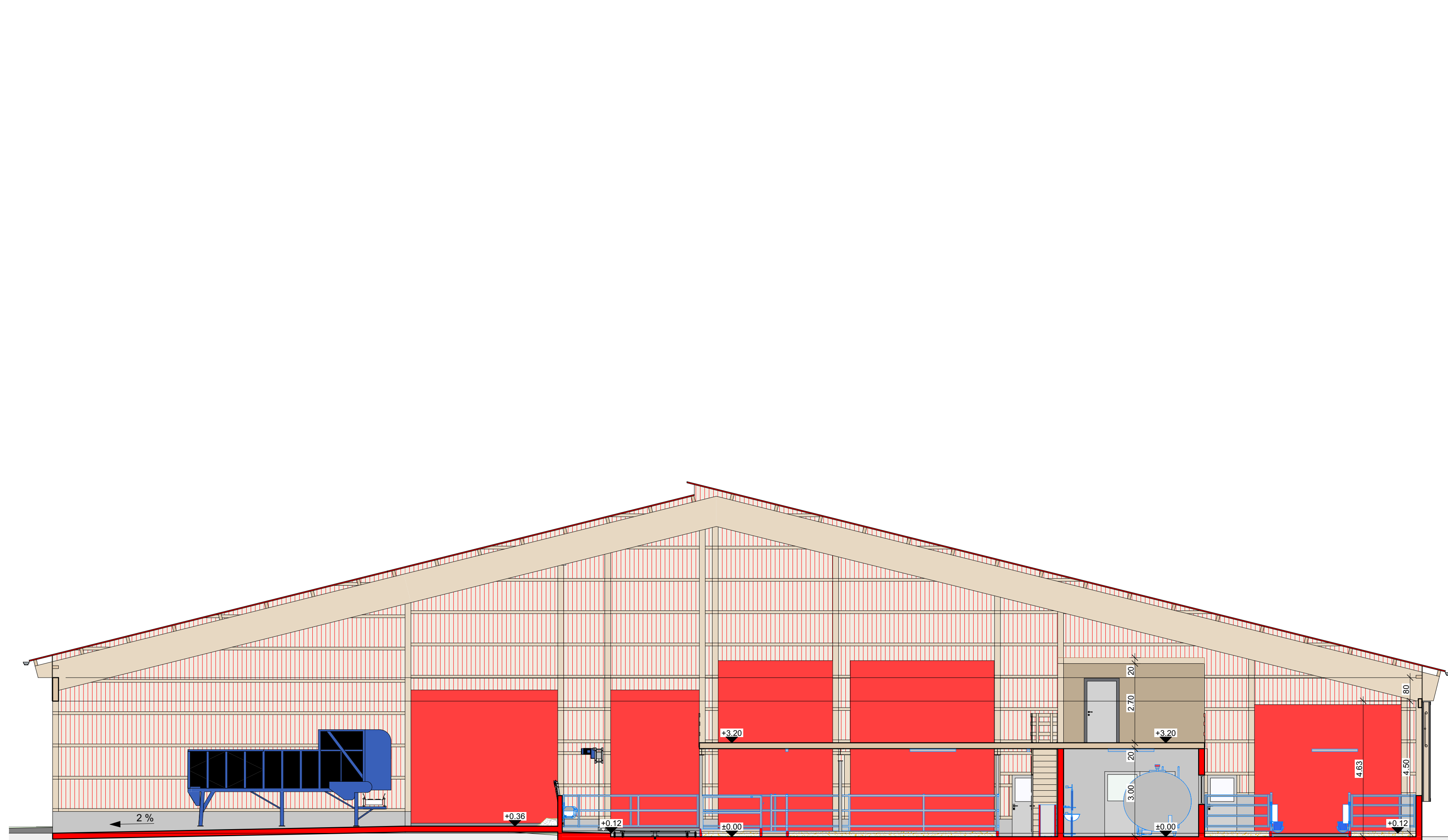
Schnitt A - A
